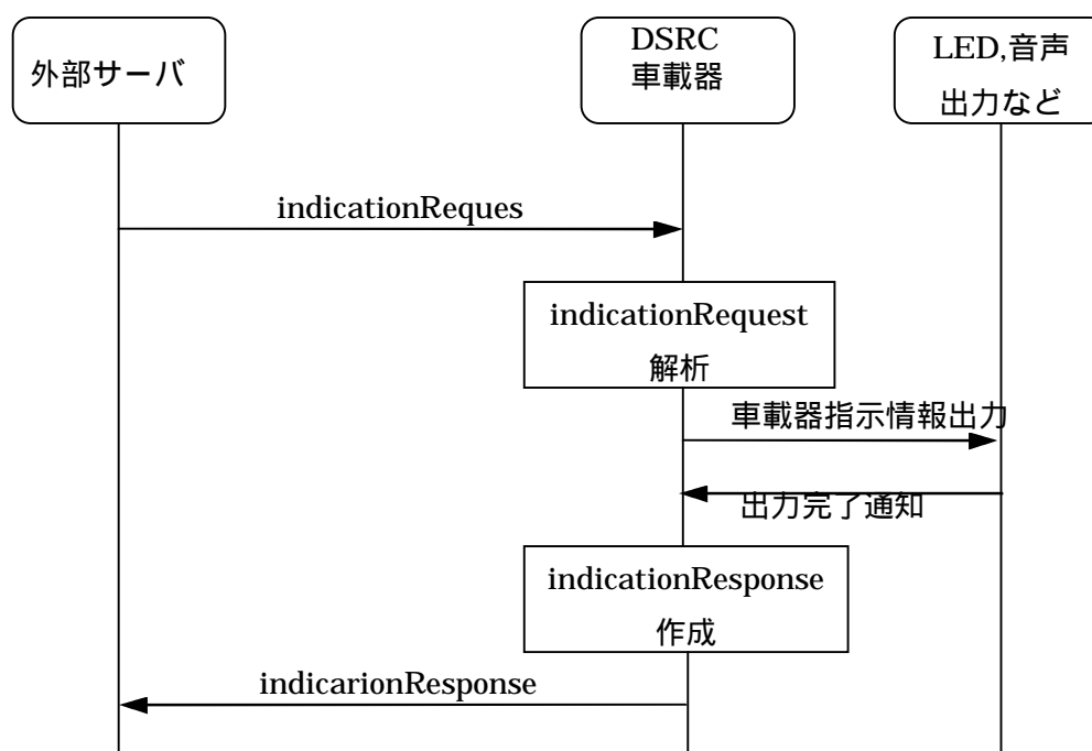
図 3.1-1 車載器への指示情報通知シーケンス例
