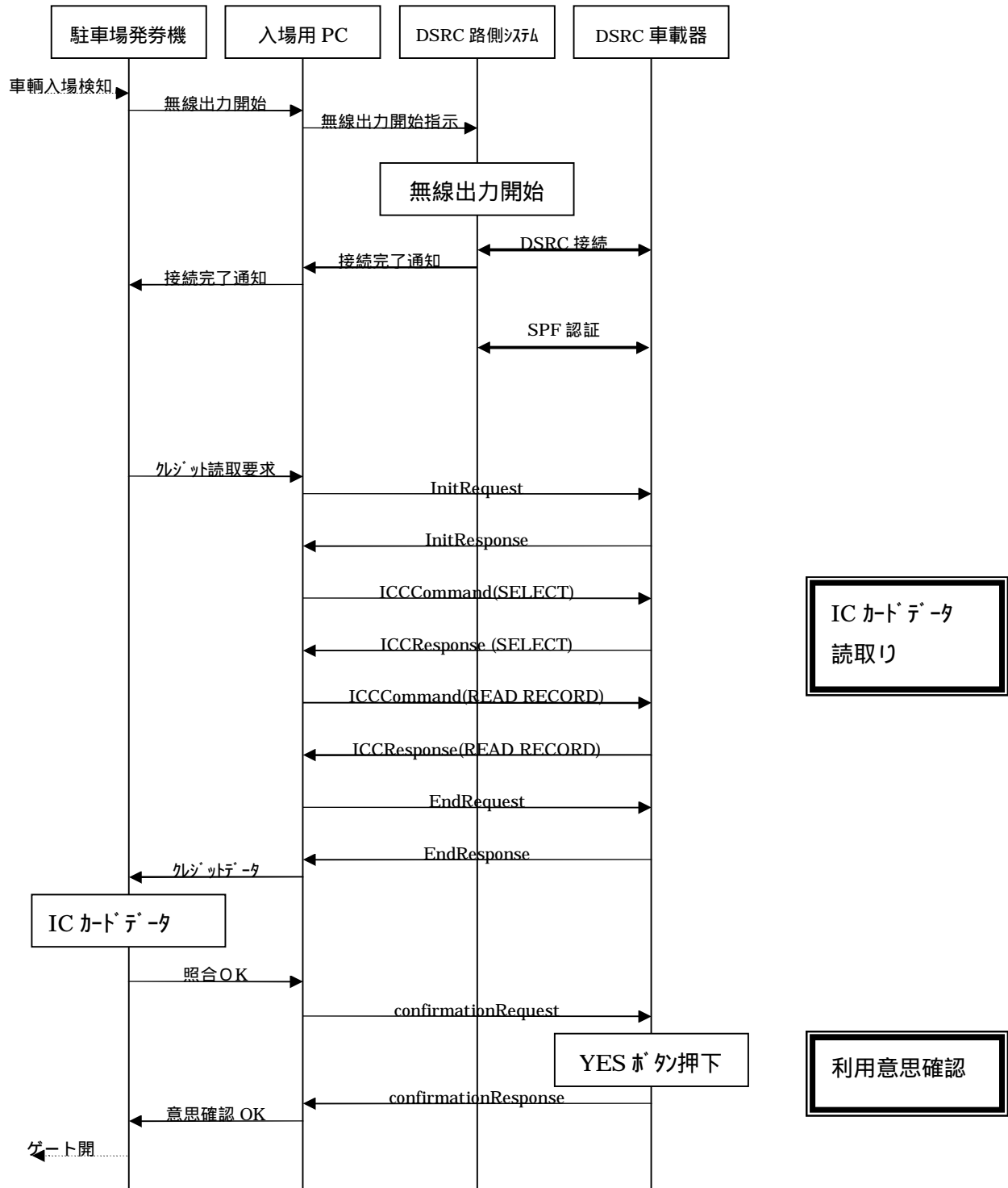
付図 C3-1 入場シーケンス
