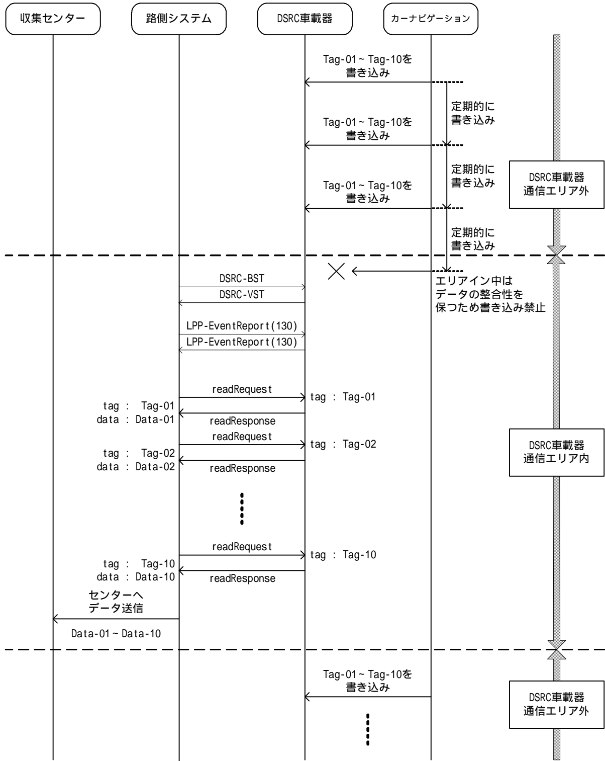
付図 D4-3 車載器管理メモリを使用した車載器アップロードシーケンス例
