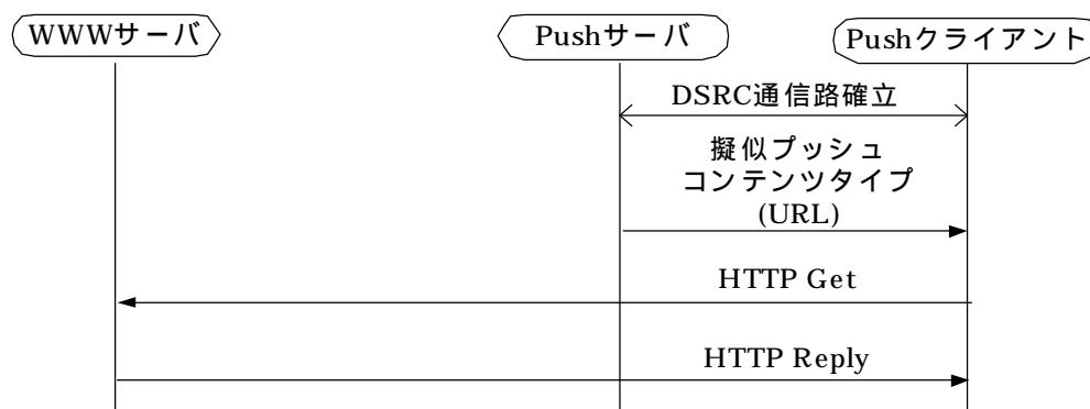
図 3.4-2 擬似プッシュの実現例
